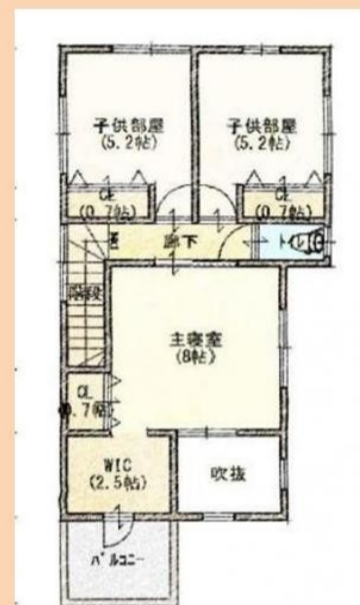
1階 (間取り) 2階
